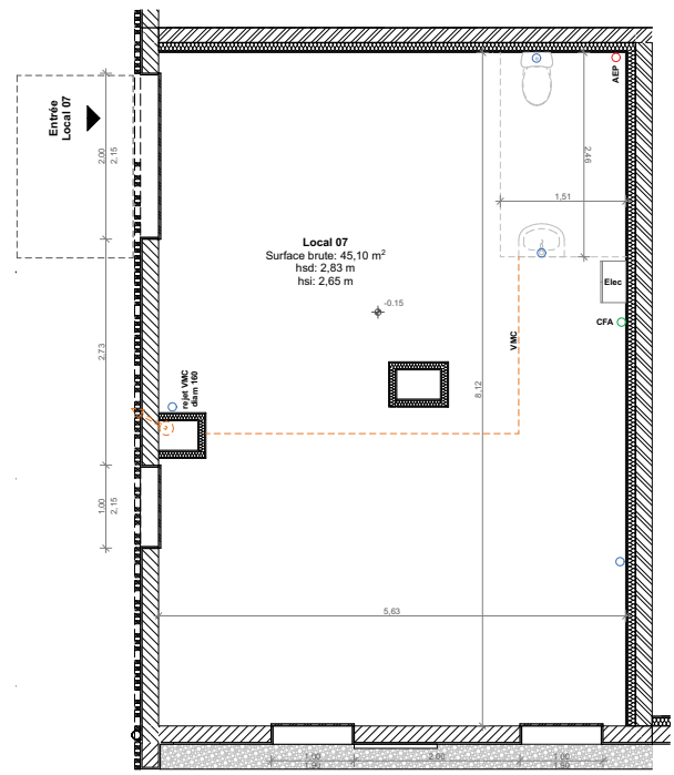
Plan du Rez-de-chausée
